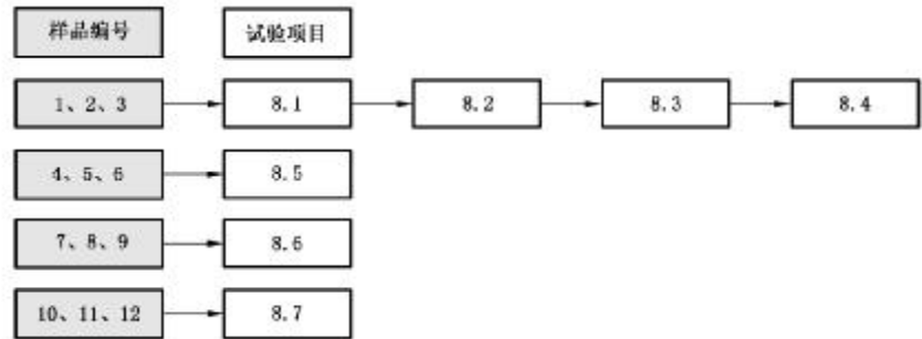
图 C.2 电池组环境安全试验顺序
