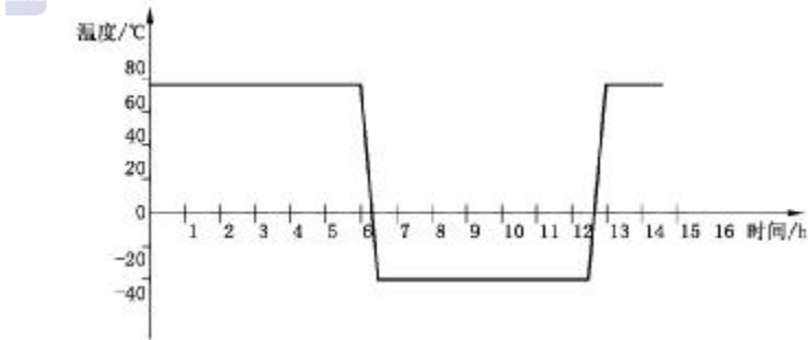
图 1 温度循环流程示意图
