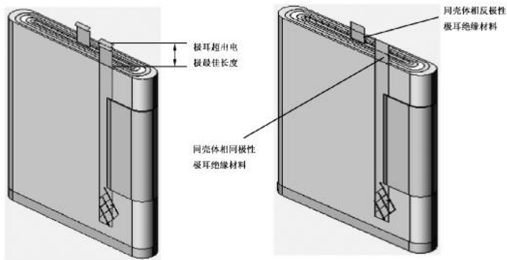
a) 电极设计中极耳最佳长度示意图 b) 电极中极耳绝缘材料放置示意图
