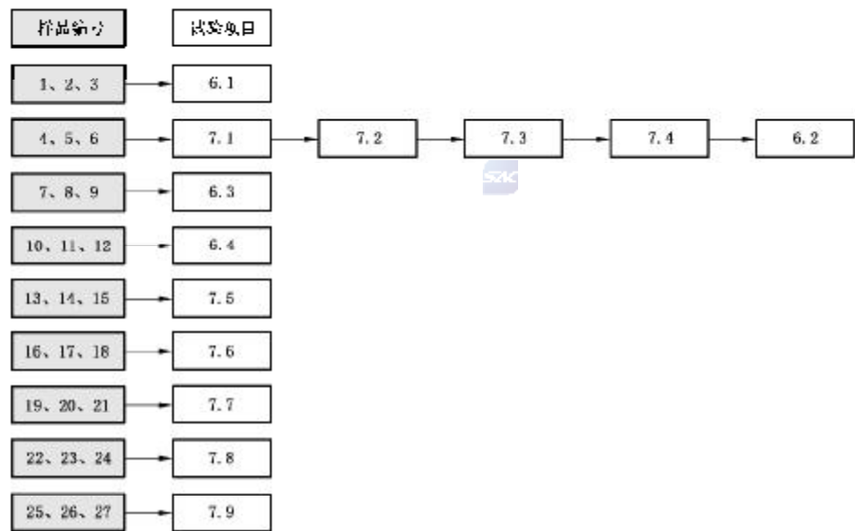
图 C.1 电池安全型式试验顺序
